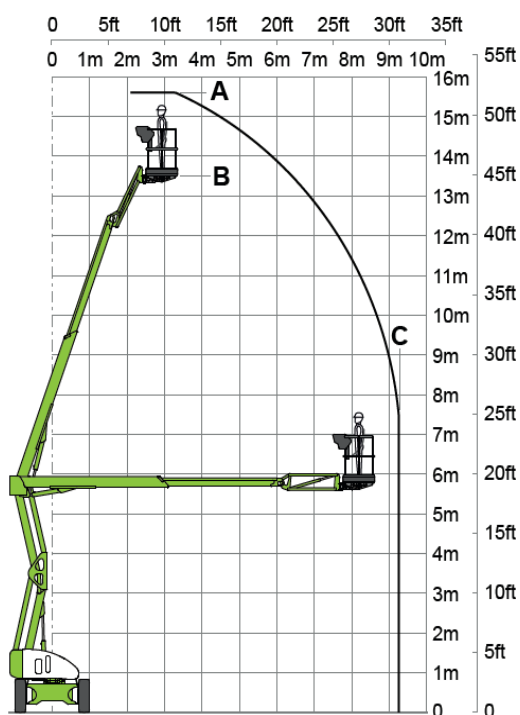
HR 15 4x4, Hybrid, Diesel + Batterie
