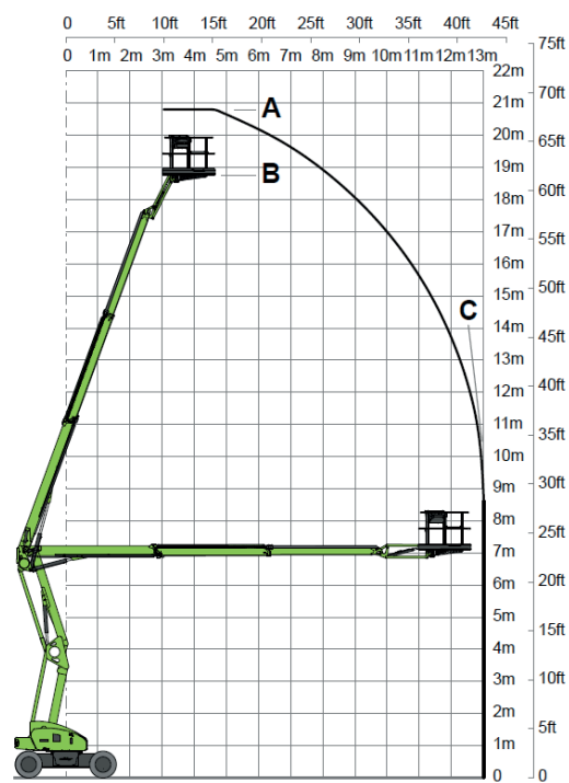
HR 21 4x4, Hybrid, Diesel + Batterie
